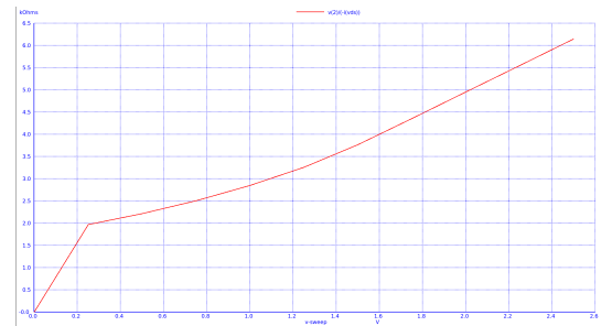
(d) Absolute resistance of nmos transistor and V_{gs} = 2.5V
